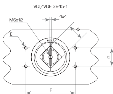
Scotch Yoke przyłącze górne
