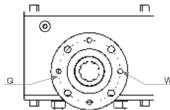
PRZYŁĄCZE POJED. KOLNIERZ ISO 5211
