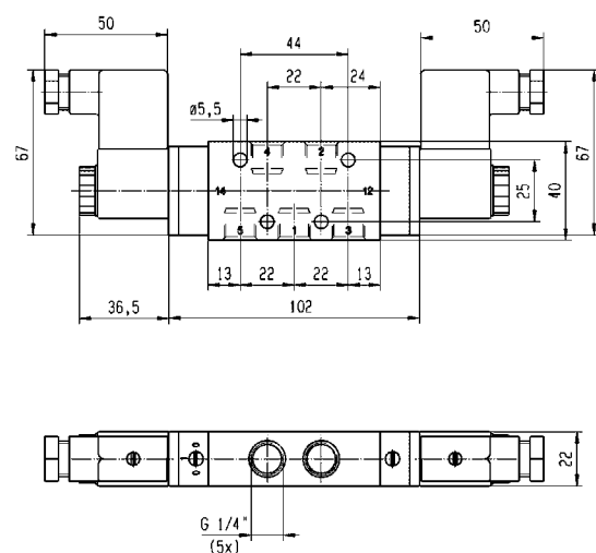
Rysunek wymiarowy 19
