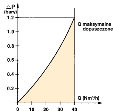
Natężenie przepływu (zawór otwarty w 100%)
