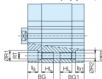
Położenie przyłącza G, J
