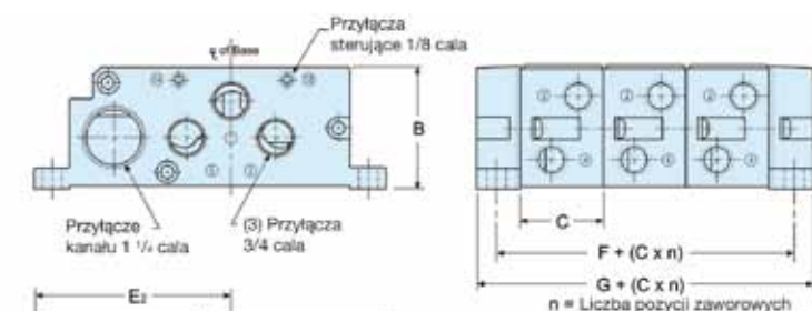
Rozdzielacz z opcjonalnym okablowaniem zbiorczym
