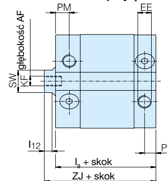
Położenie przyłącza G
