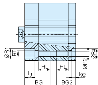
Położenie przyłącza G
