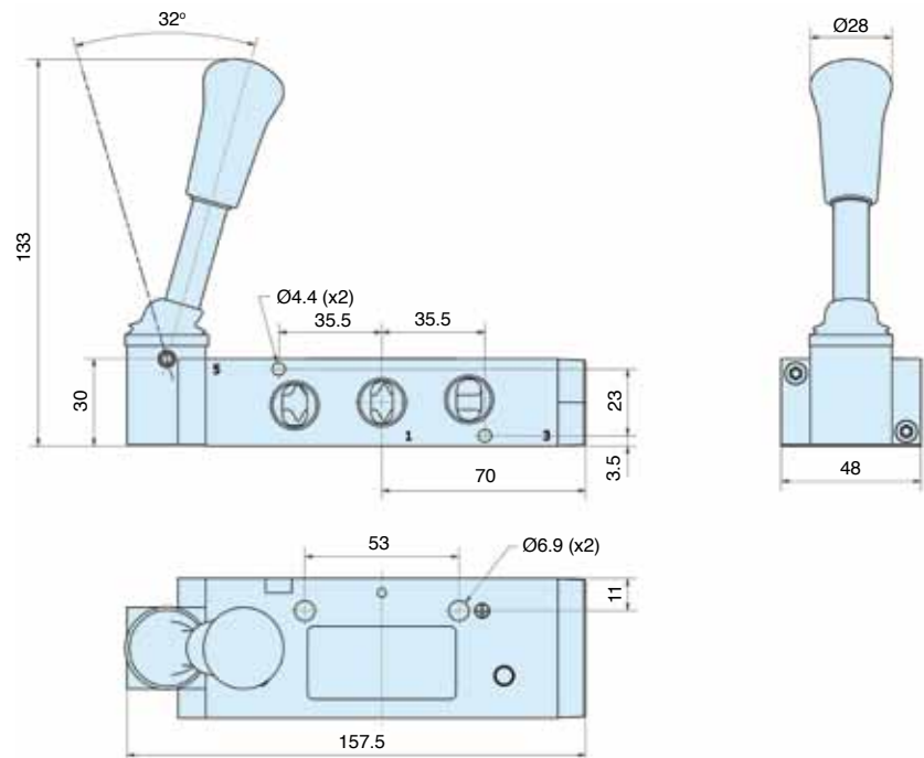
P2LCX – Zawory sterujące 5/3 uruchamiane dźwignią
