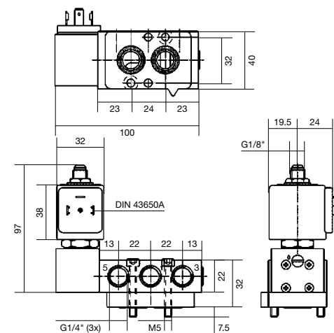
Rysunek wymiarowy 5
