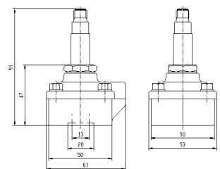
Rysunek wymiarowy Nr 6
