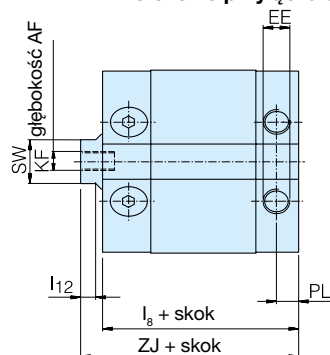
Położenie przyłącza J
