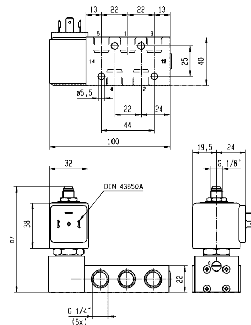
Rysunek wymiarowy 20
