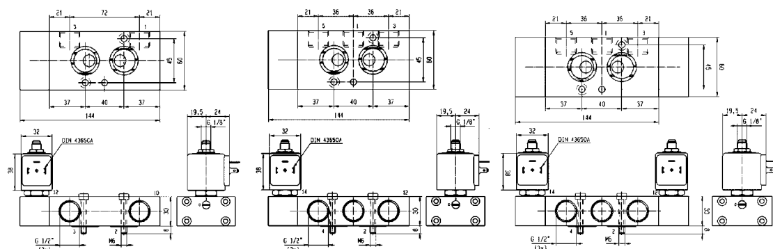
Rysunek wymiarowy 13
