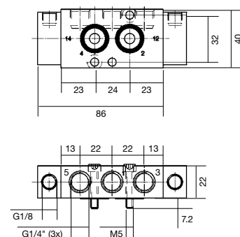
Rysunek wymiarowy 9
