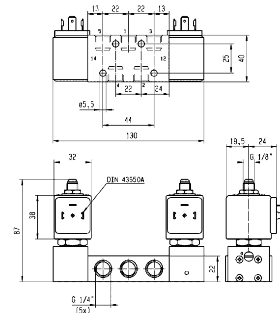
Rysunek wymiarowy 21
