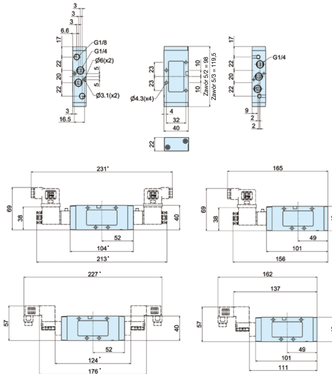
P2LBX... wszystkie Zawory 5/2 i 5/3
