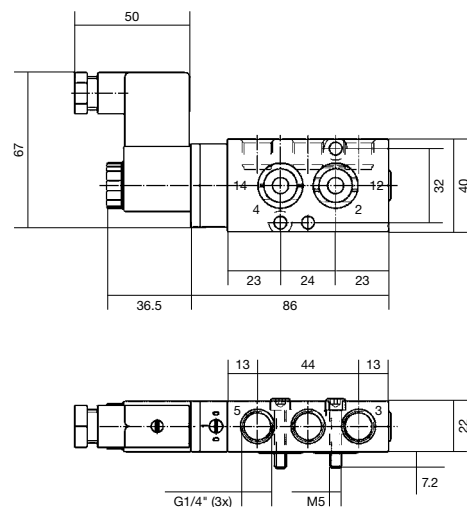
Rysunek wymiarowy 4
