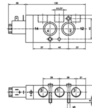
Rysunek wymiarowy 11
