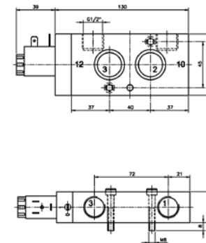
Rysunek wymiarowy 10
