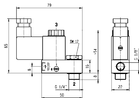
Rysunek wymiarowy 27
