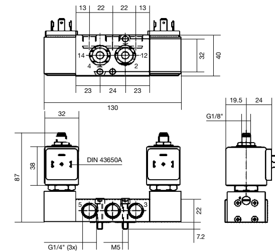
Rysunek wymiarowy 6
