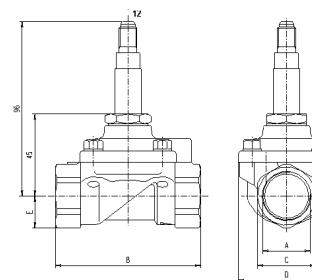
Rysunek wymiarowy Nr 4
