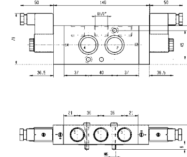
Rysunek wymiarowy 12
