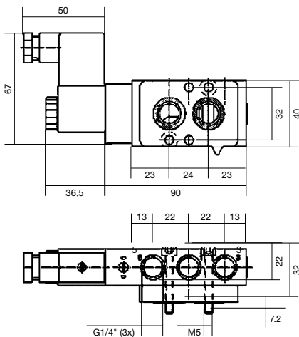
Rysunek wymiarowy 3
