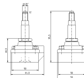
Rysunek wymiarowy Nr 6
