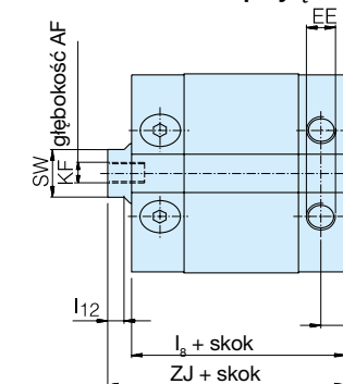
Położenie przyłącza J
