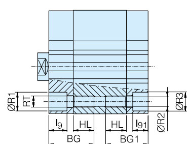
Położenie przyłącza H
