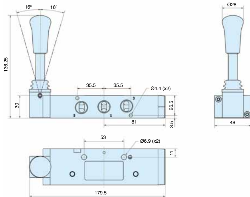
P2LCX – Zawory sterujące 5/3 uruchamiane dźwignią
