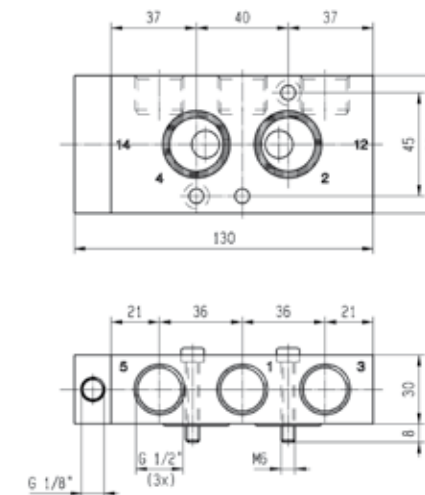
Rysunek wymiarowy 17
