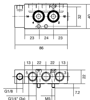
Rysunek wymiarowy 8
