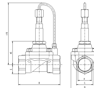
Rysunek wymiarowy Nr 2
