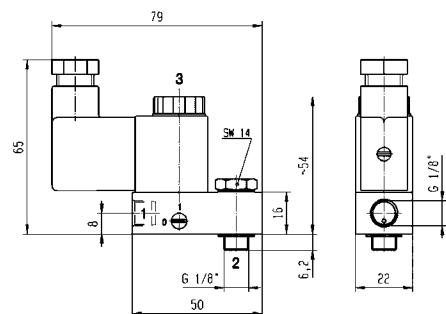
Rysunek wymiarowy 26
