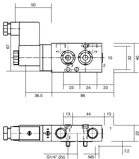
Rysunek wymiarowy 3
