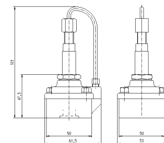
Rysunek wymiarowy Nr 7
