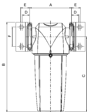
Zestaw DPI P3TKA00RQ
