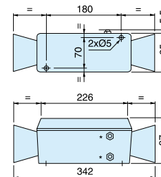
PXP-C111 i PXP-D121
