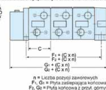
Rozdzielacz z opcjonalnym okablowaniem zbiorczym
