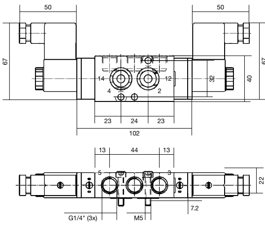
Rysunek wymiarowy 4
