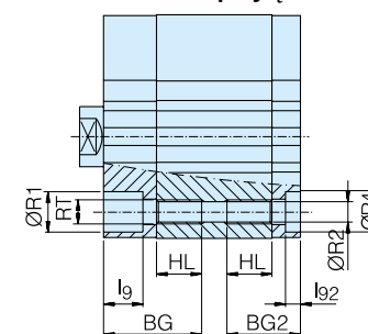
Położenie przyłącza H
