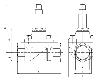
Rysunek wymiarowy Nr 3
