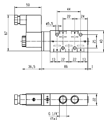
Rysunek wymiarowy 18
