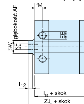
Położenie przyłącza H
