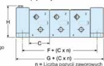
Rozdzielacz z opcjonalnym okablowaniem zbiorczym
