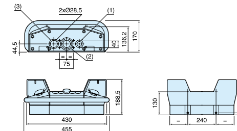
PXP-S111 i PXP-S121
