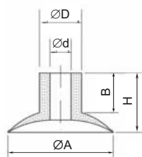
PVG 4 ÷ 22
