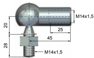
2-M14 Winkelgelenk • Angle joint Joint à angle • Snodo angolare Charnela articulada
