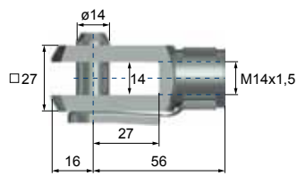
3-M14 Gabelkopf • Female rod clevis Embout à rotule (femelle) Forcella femmina Charnela hembra
