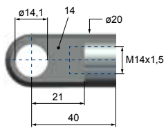
1-M14 Gelenkauge • Male rod clevis Tête de chape (male) Attacco a cerniera maschio Charnela macho
